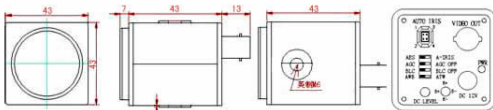
型号: VS-908HC
