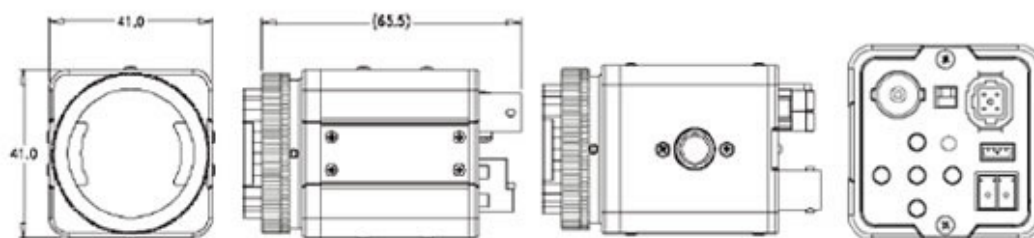
型号: VS-906HC
